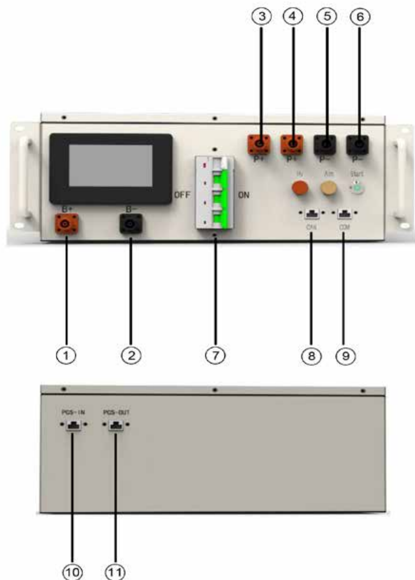
Fig. 3-4 HV Box interface
